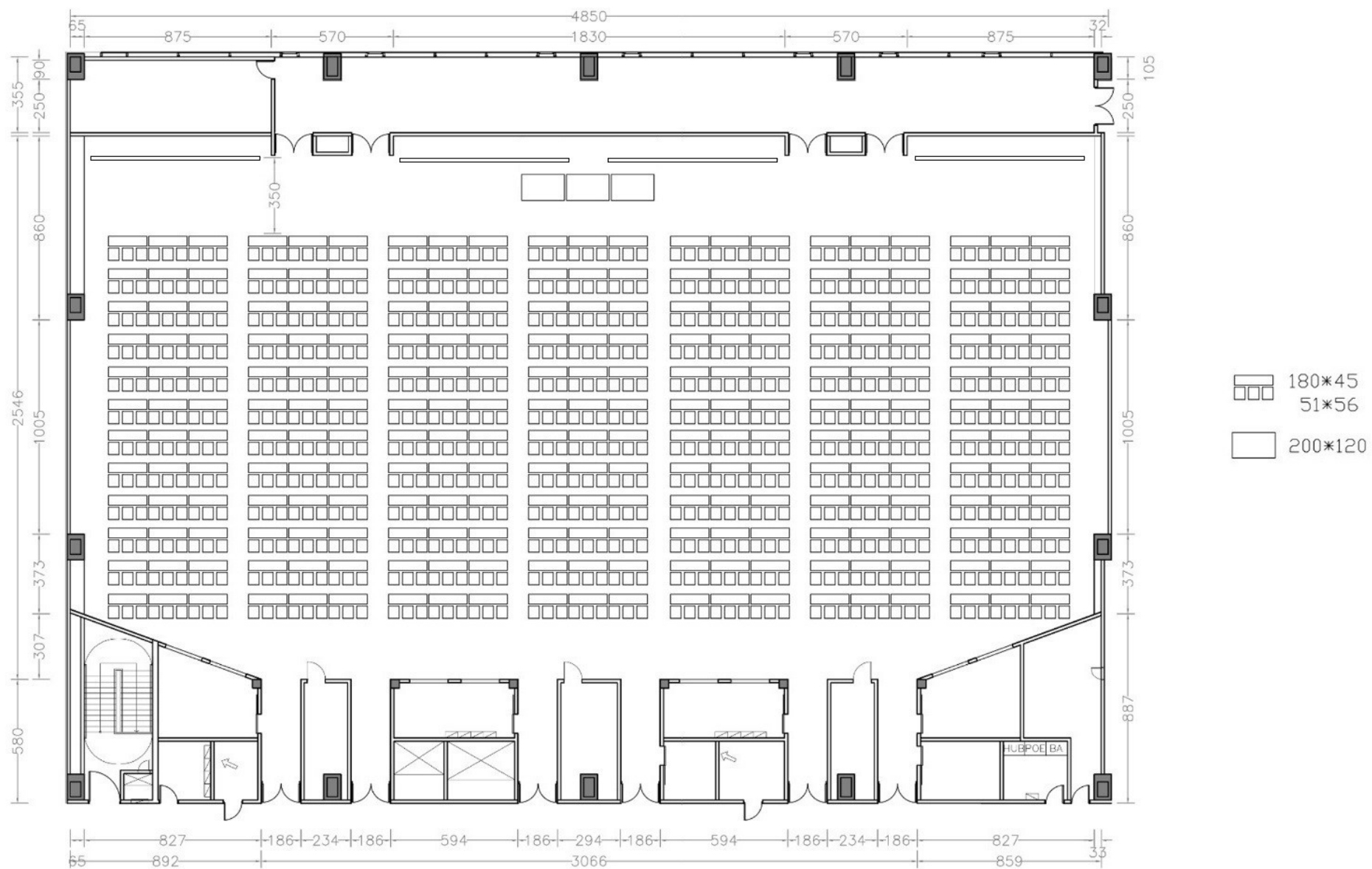
@樓層三大員廳 (教室型756人)
